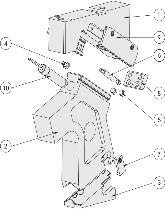
构成零件 Component parts
