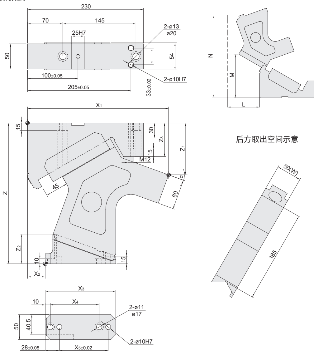
斜楔结构图 Diagram of Cam Structure
